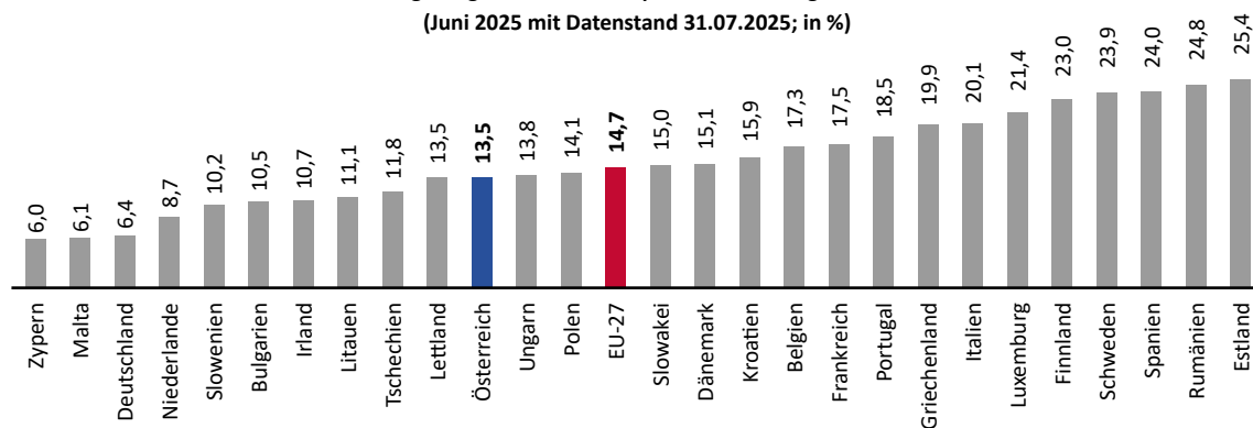
Saisonbereinigte Jugendarbeitslosenquoten im EU-Vergleich laut Eurostat (Juni 2025 mit Datenstand 31.07.2025; in %)
