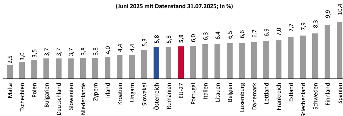
Saisonbereinigte Arbeitslosenquoten im EU-Vergleich laut Eurostat (Juni 2025 mit Datenstand 31.07.2025; in %)
